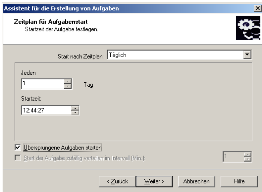
Abb. 24: Täglicher Aufgabenstart
