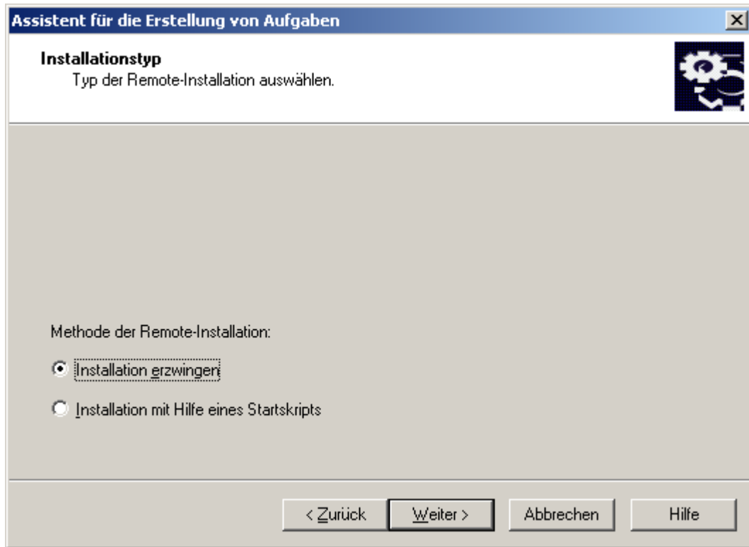
Abb. 15: Installationsmethode auswählen
