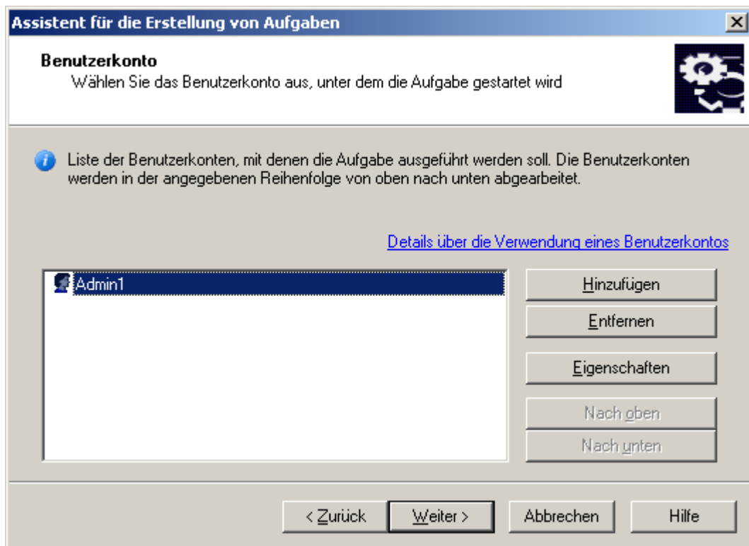
Abb. 23: Benutzerkonto auswählen
