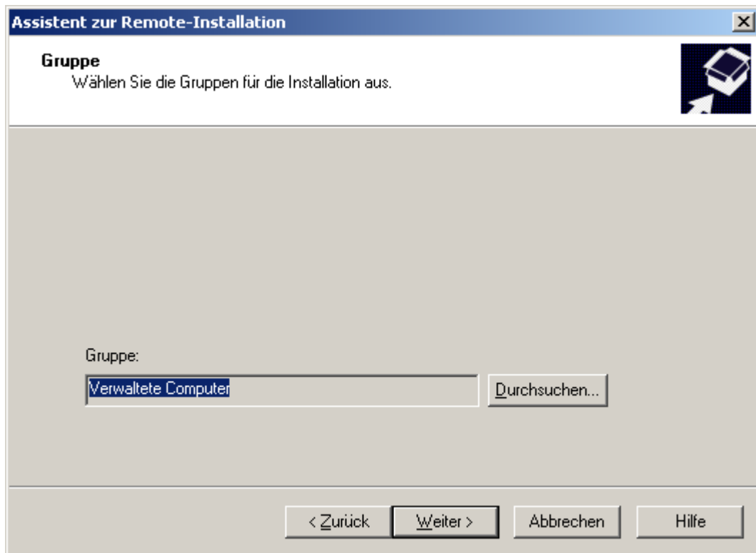
Abb. 37: Gruppe auswählen
