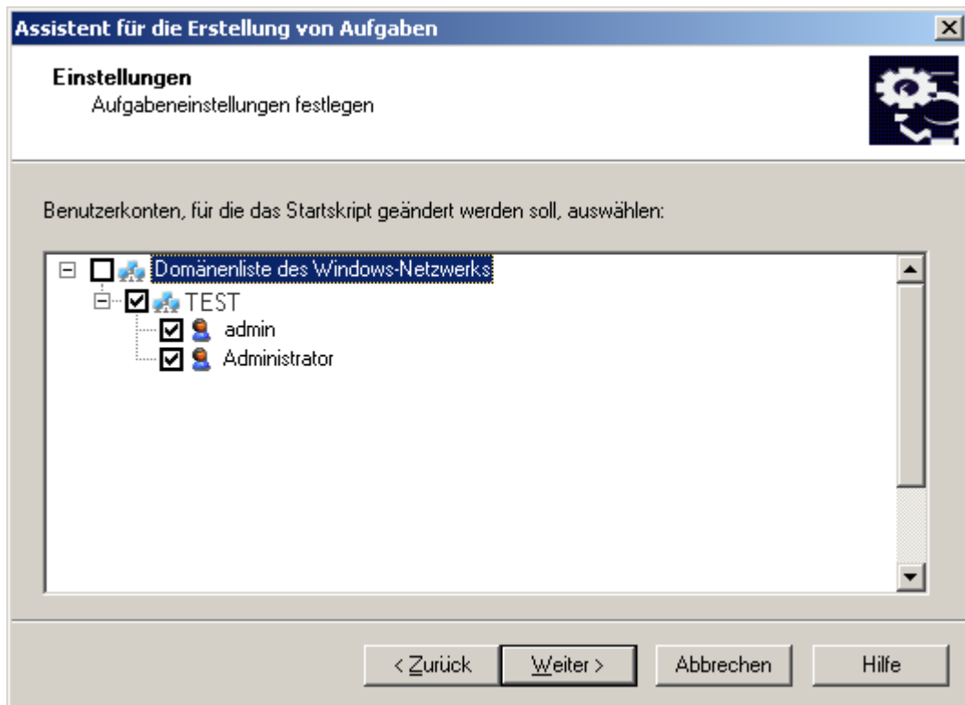
Abb. 28: Benutzerkonten auswählen
