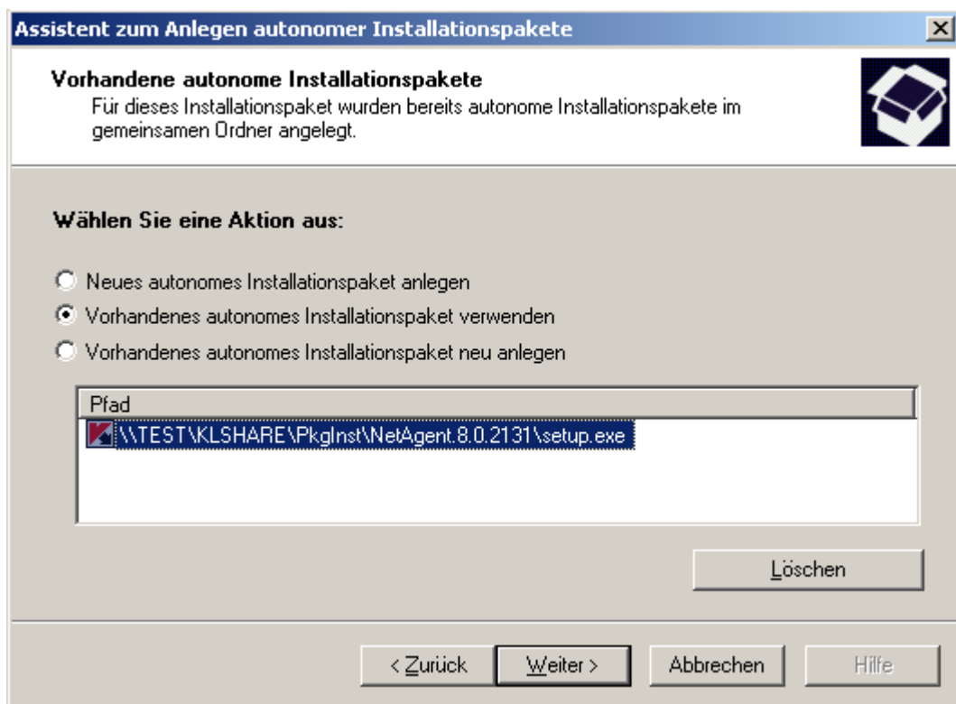
Abb. 64: Aktion auswählen
