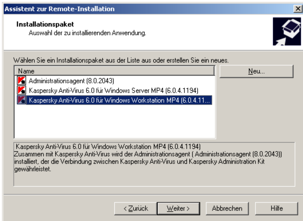
Abb. 35: Installationspaket auswählen
