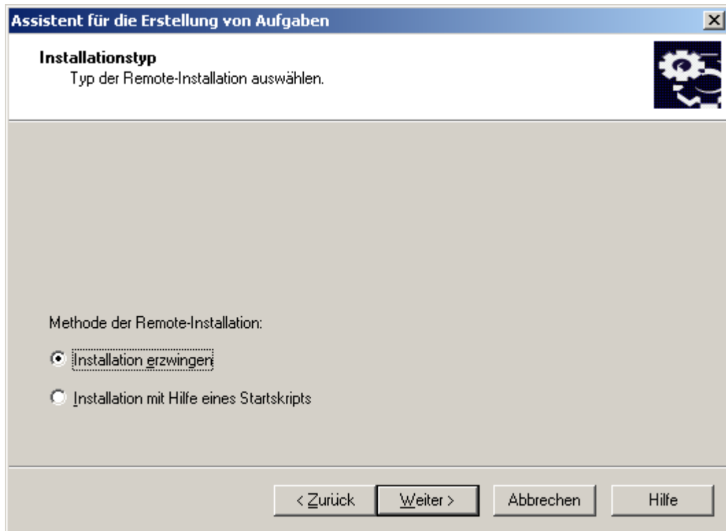
Abb. 27: Installationsmethode auswählen
