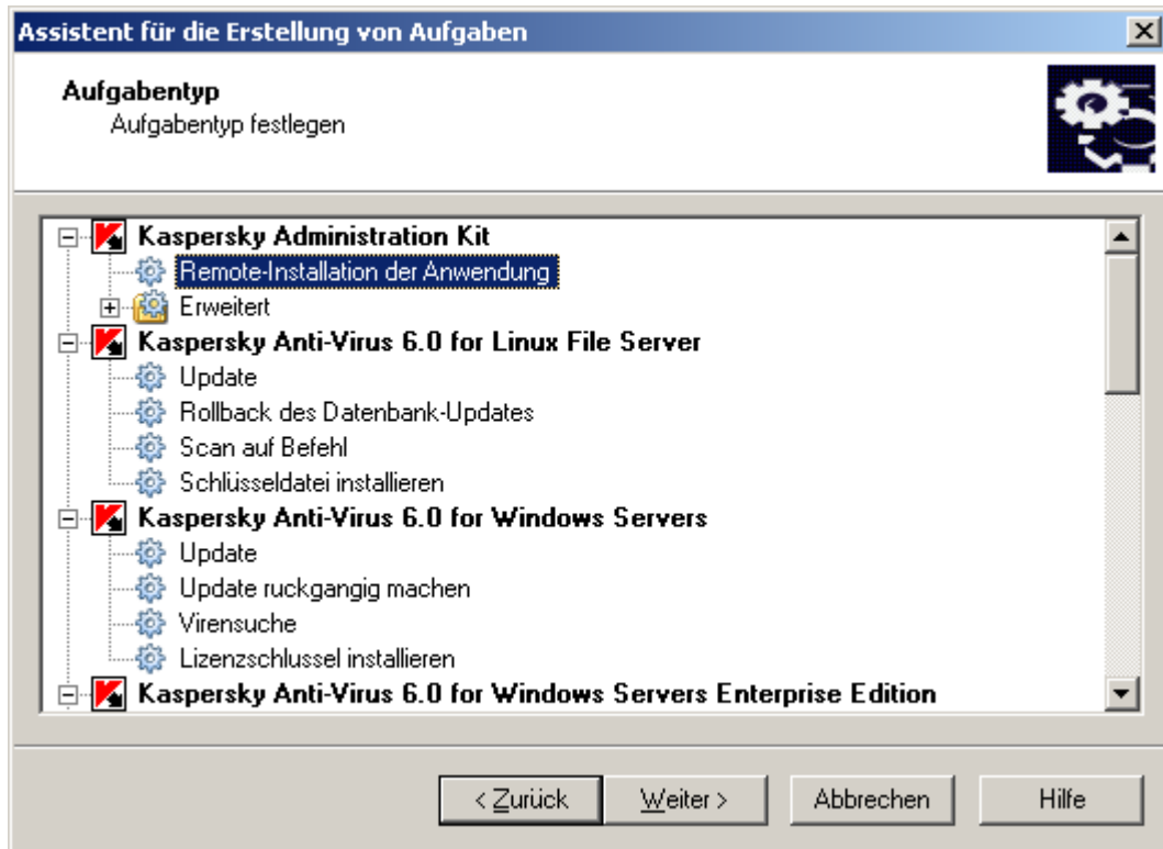
Abb. 25: Aufgabenart festlegen
