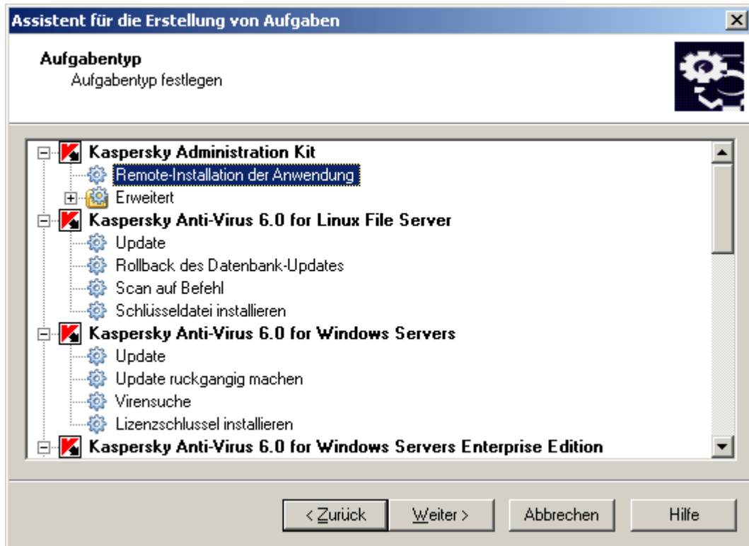
Abb. 13: Aufgabenart festlegen
